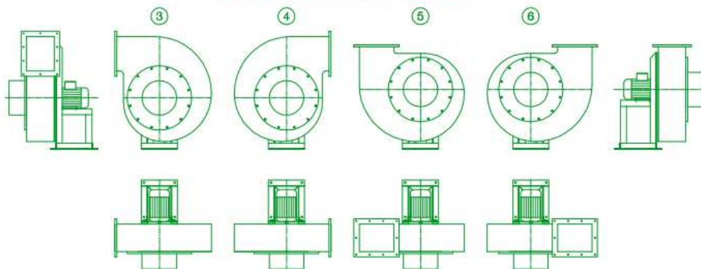
מצב בית המפוח במבט מכיוון היניקה
